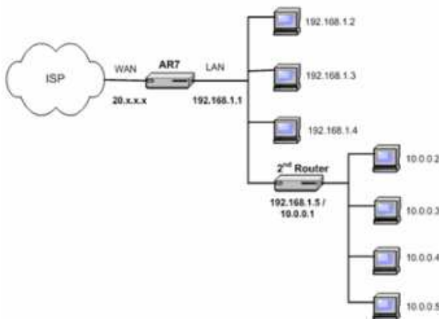
Statické směrování – LAN s podsítí
