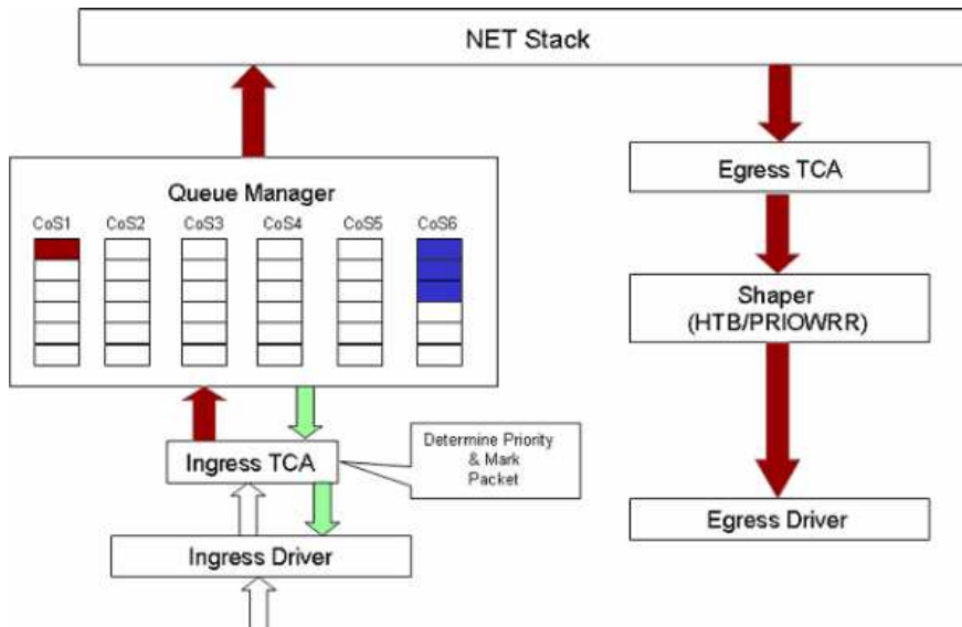
Schéma toku QoS routeru
